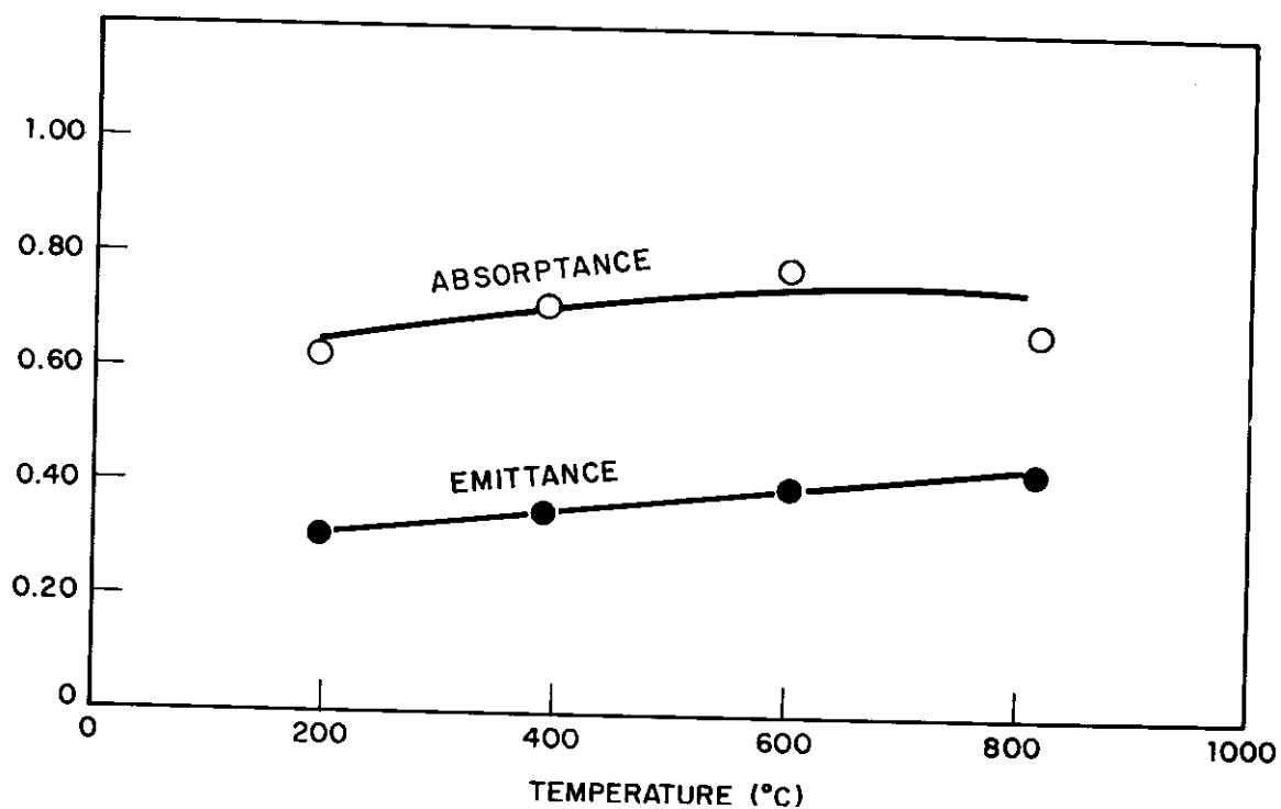
Fig. 19 Tungsten carbide on Armco iron.
